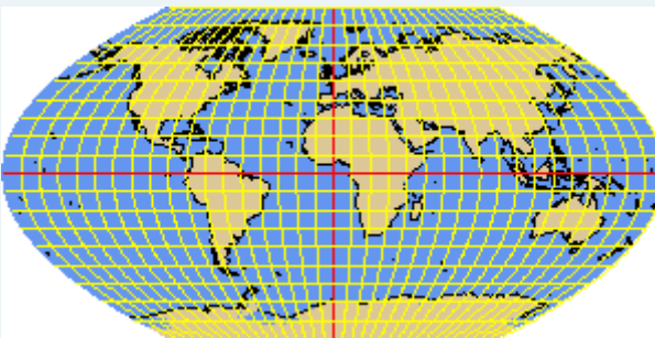
PUTNINS3P parabolic
